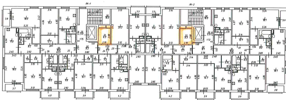
План 5 этажа л. 272
