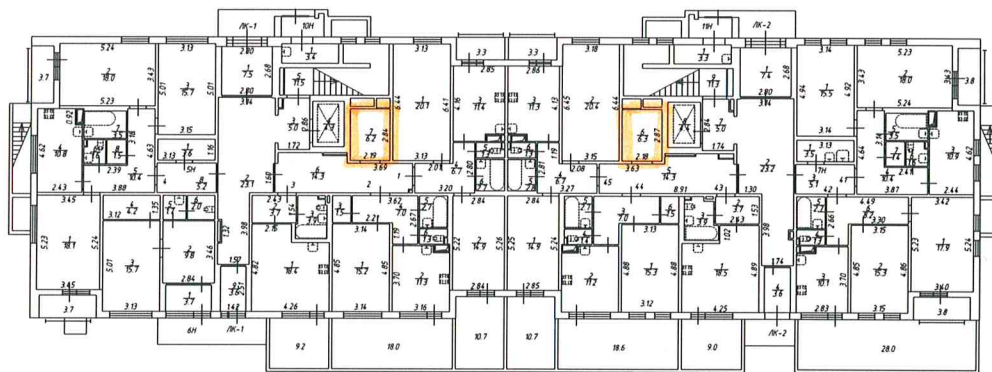
План 1 этажа Л-283
